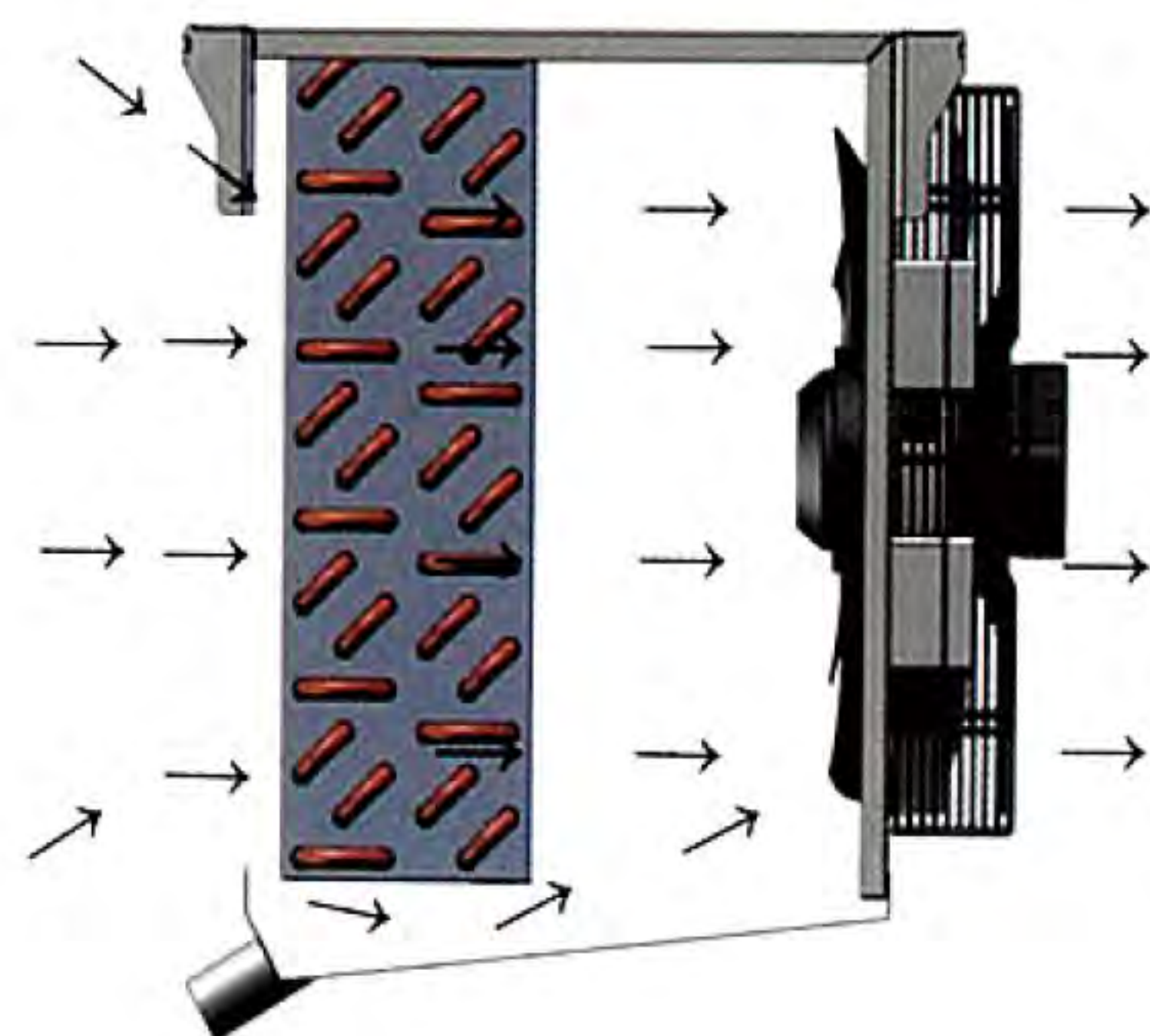
无挡风板 w/o windshield
